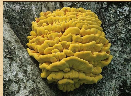
Laetiporus sulphureus , Серно-жёлтый трутовик
