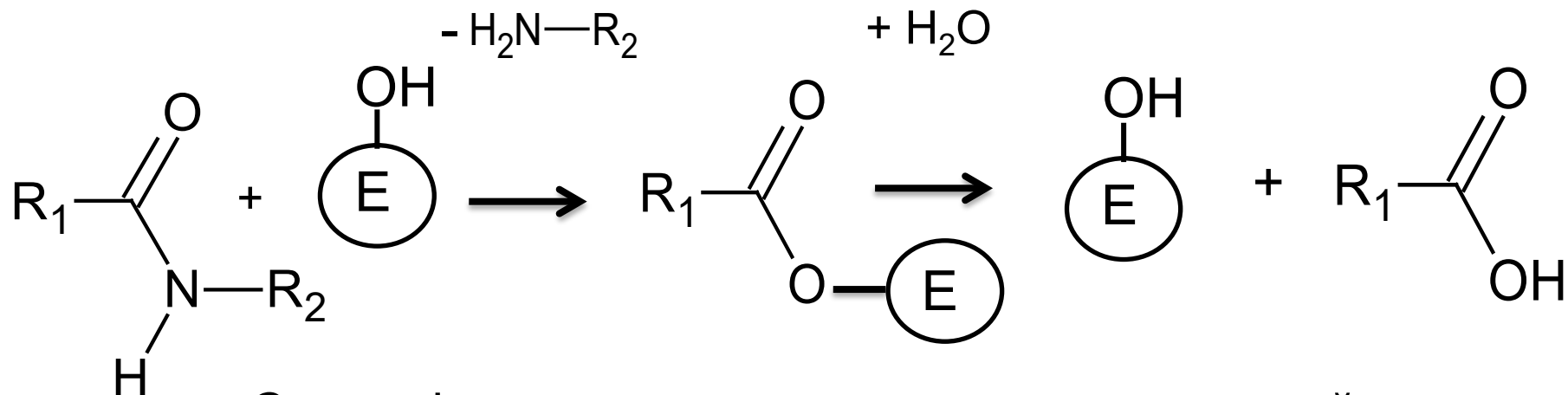
Схема ферментативного гидролиза пептидной связи
