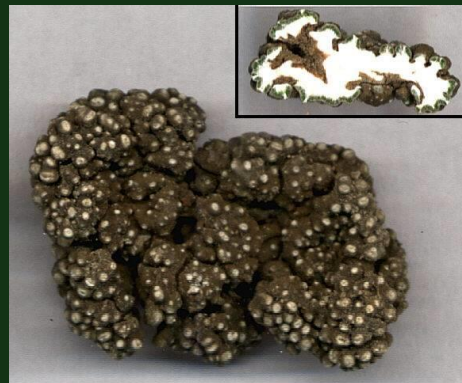
Aspicilia vagans
