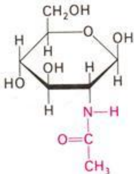
N-ацетилглюкозамин (NAG)
