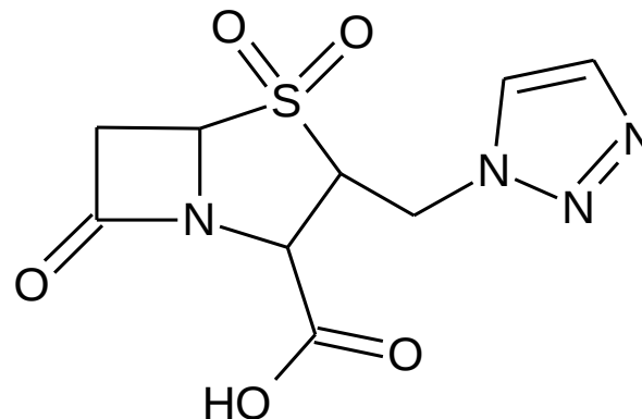
тазобактам
