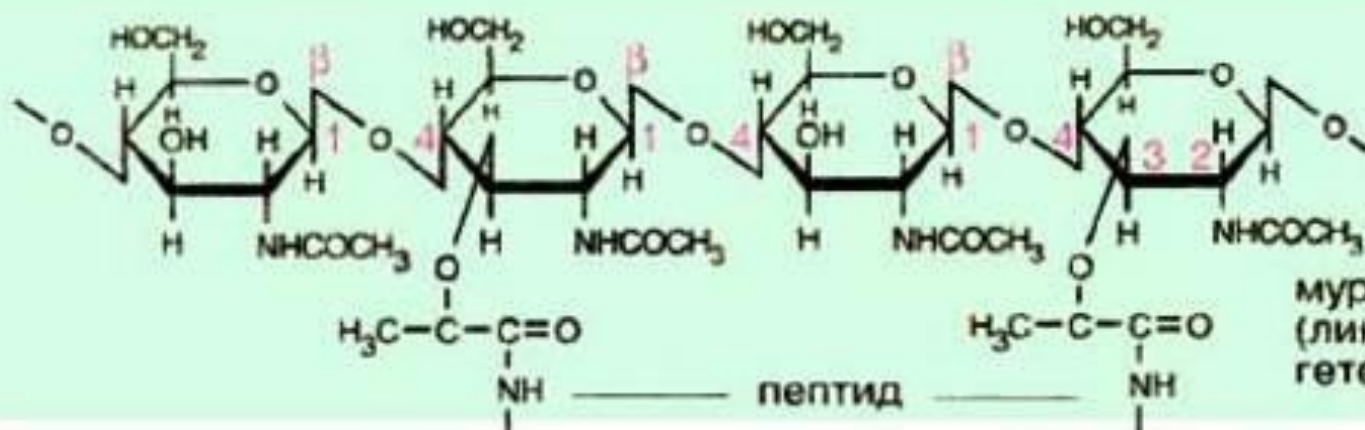
N-ацетилглюкозамин (NAG)
