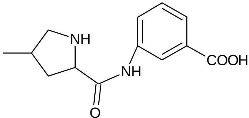
Эртапенем
