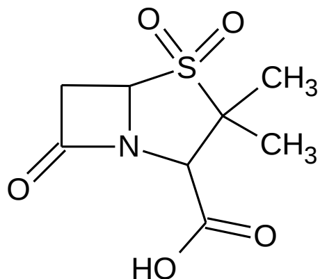
сульбактам
